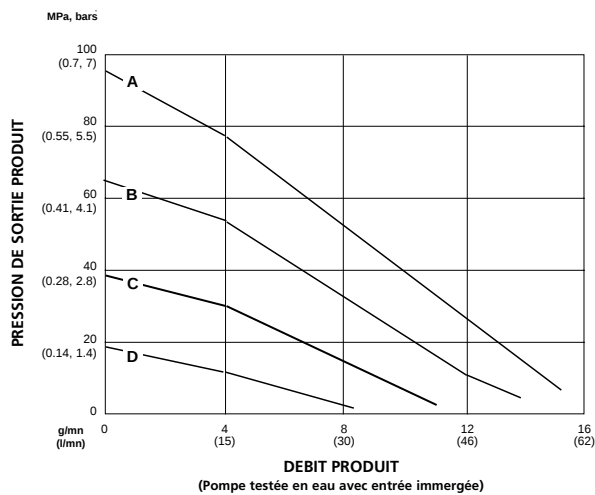
Pression produit
