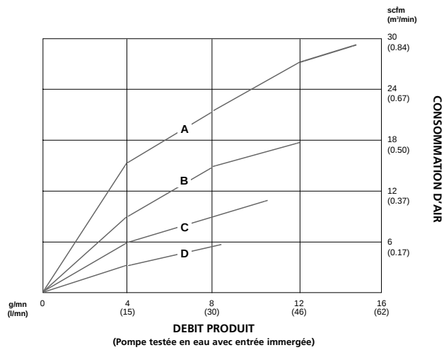
Consommation d'air
