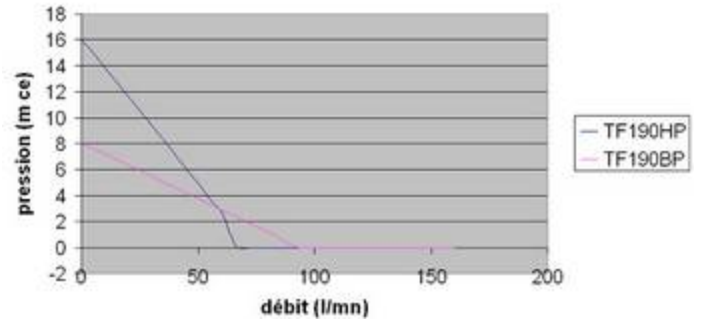
POMPE VIDE FUT TECHNI-FLOW TF190HP/TF190BP
