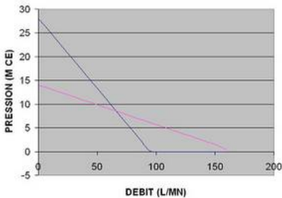
POMPE VIDE FUT TECHNI-FLOW TF280 HP/TF280BP
