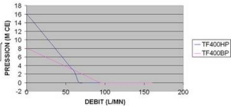
POMPE VIDE FUT TECHNI-FLOW TF400HP/TF400BP
