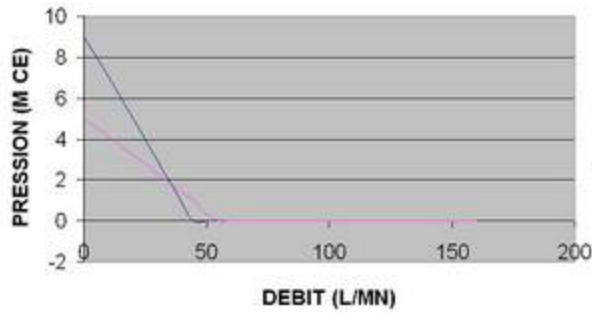
POMPE VIDE FUT TECHNI-FLOW TF280 HP/TF280BP
